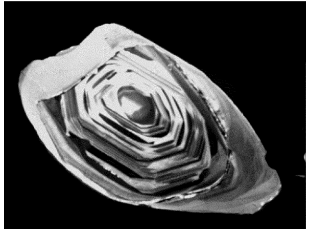
图3 具二期生长历史锆石的阴极发光 CL 图像
