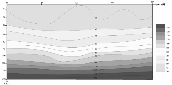
图 5 40 线电阻率测深法视电阻率等值线断面图
