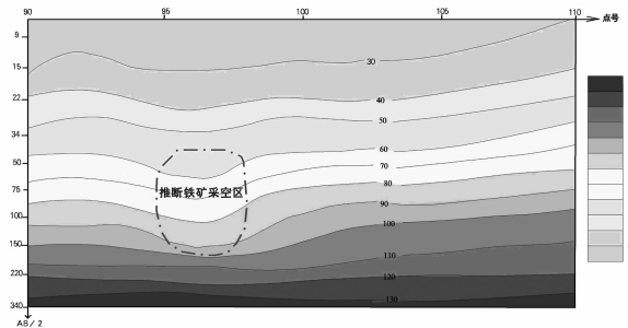
图 2 10 线电阻率测深法视电阻率等值线断面图
