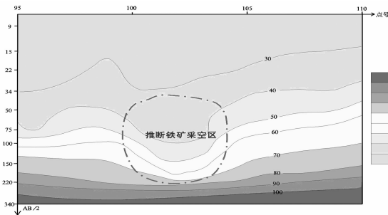
图 4 20 线电阻率测深法视电阻率等值线断面图 根据调查和结合电法、磁法资料,推断认为采空区范围与磁力线 600 nT 异常范围相吻合,深约 40 ~ 55 m,采空区影响范围约 7 500 m 2 。
