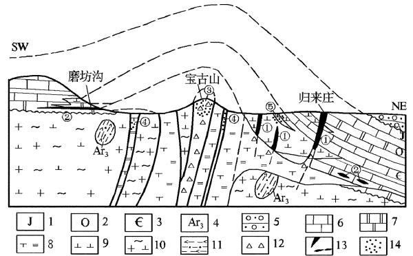
图5 归来庄金矿田矿床组合模式图
