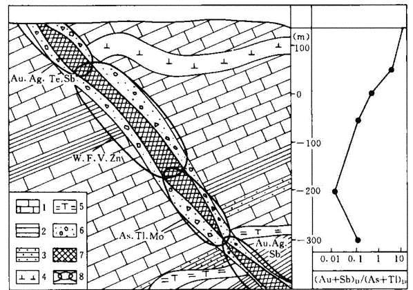
图6 归来庄金矿床地球化学矿体定位模型
