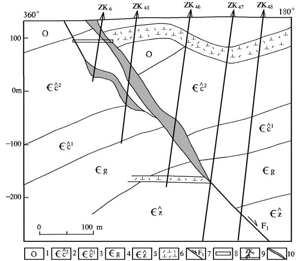
图3 平邑归来庄金矿30线地质剖面图
