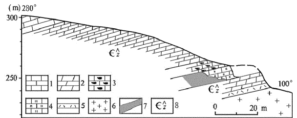
图4 平邑磨坊沟金矿地质剖面图
