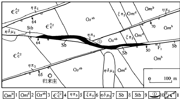
图2 平邑归来庄金矿地质略图
