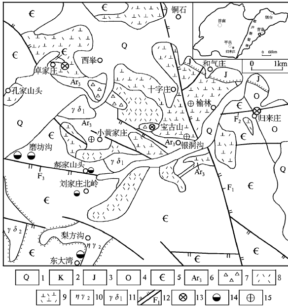
图1 平邑铜石地区地质矿产略图
