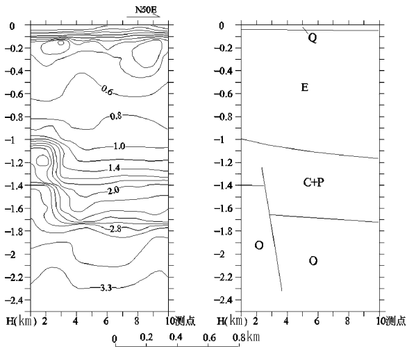
图4 III剖面 MT 二维反演电阻率断面图及解释推断成果图
