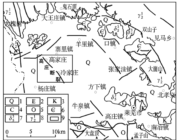
图 1 莱芜市冷家庄地区地质简图
