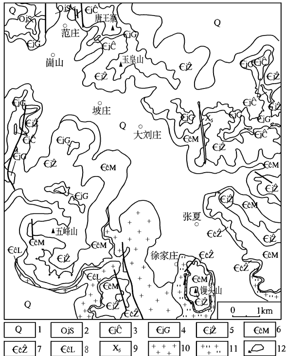
图 1 张夏-崮山地区区域地质略图
