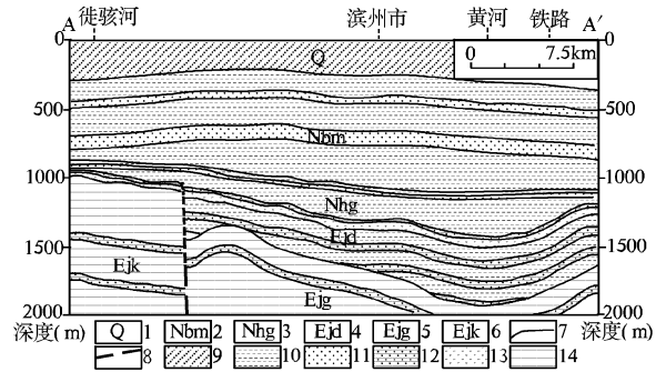
图 2 滨州市城区地热地质剖面图
