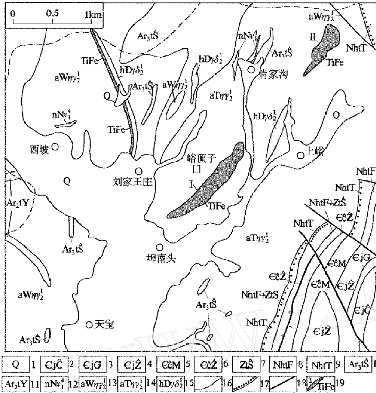
图 1 莒县天宝钛铁矿矿区地质图
