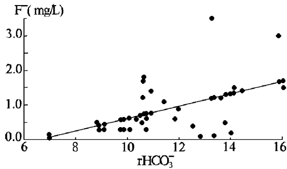
图 5 氟含量与总碱度相关散点图
