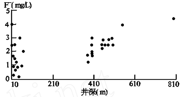
图 1 地下水氟含量与井深关系散点图
