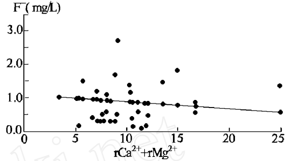
图 6 氟含量与总硬度相关散点图
