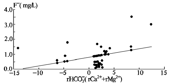
图 7 氟与 [rHCO_3^- - (rCa^{2+} + rMg^{2+})] 相关散点图
