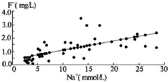
图 2 氟含量与钠含量关系散点图
