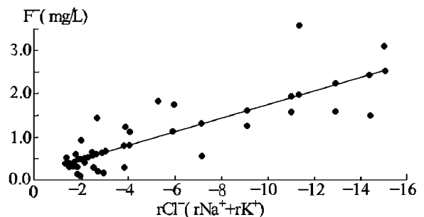
图 8 氟含量与 [rCl^- - (rNa^+ + rK^+)] 相关散点图
