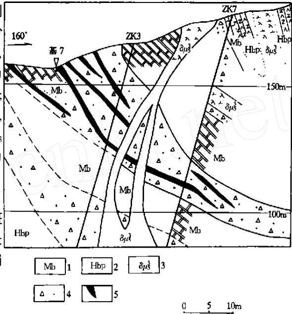
图2 土堆地段第七勘探线剖面图(示层间滑动构造带)
