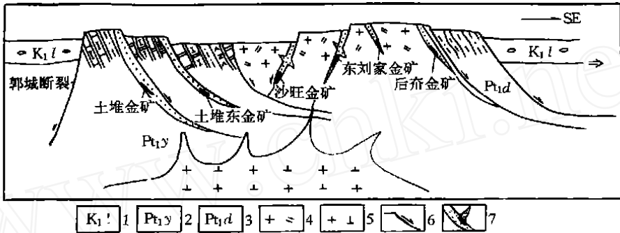
图 3 东刘家地区金矿成矿模式图
